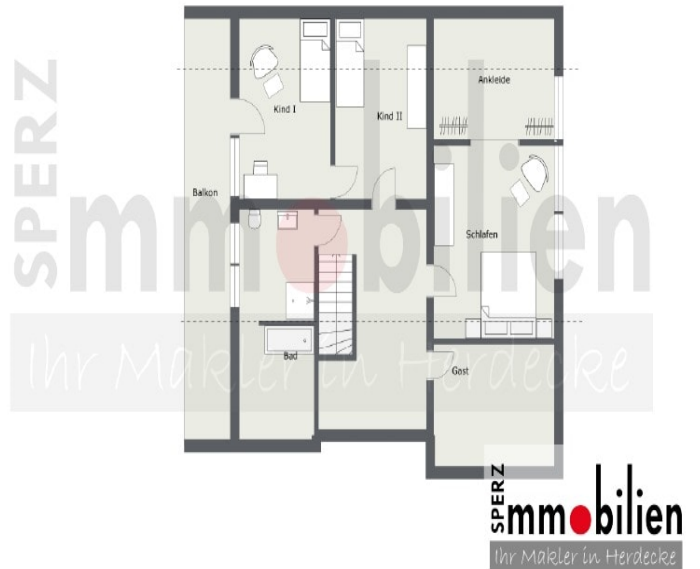
Zweifamilienhaus Obergeschoss
